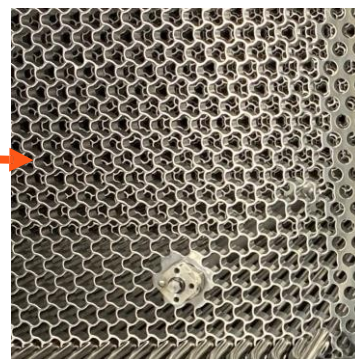
Figure 39 : Usinage trifolié
